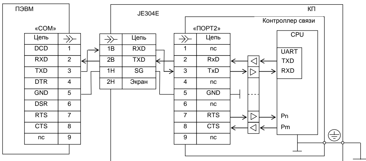
Рисунок 5 – Схема подключения контроллера связи SM2xx к ПЭВМ через клеммник защиты
