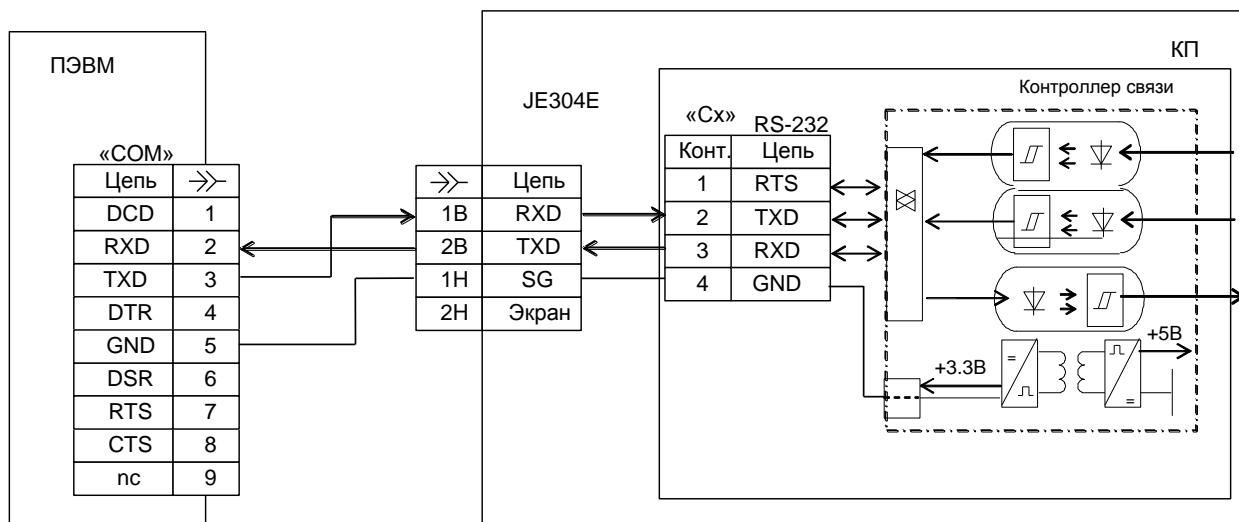
Рисунок 4 – Схема подключения контроллера связи BNSxx к ПЭВМ через клеммник защиты
