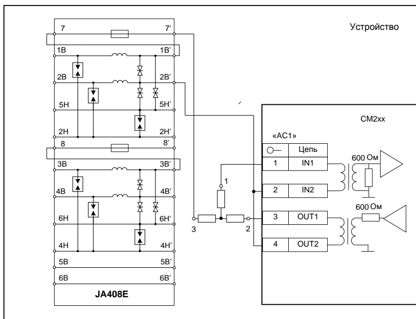
Рисунок 29 – Пример подключения контролера CM2xx к двухпроводной линии связи C1-T4
