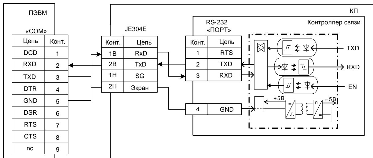
Рисунок 6 – Схема подключения контроллеров BQ3xx, SK2xx к ПЭВМ через клеммник защиты
