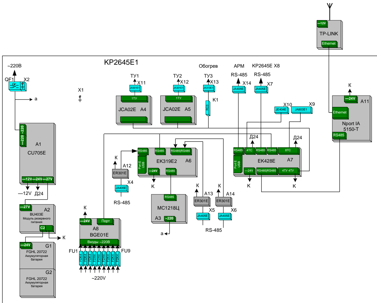
Рисунок 31 – Структурная схема устройства КР2645Е1
