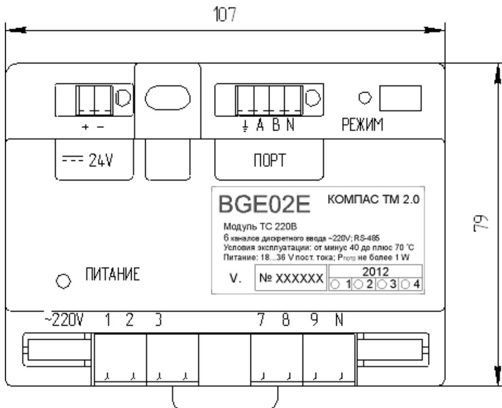
Рисунок 1 – Функциональная схема клеммника и назначение контактов его разъемов для внешних подключений
